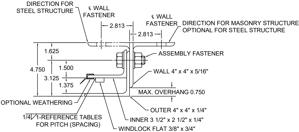
GUIDE ASSEMBLY TYPE 445 SCALE: 3" = 1'-0"
